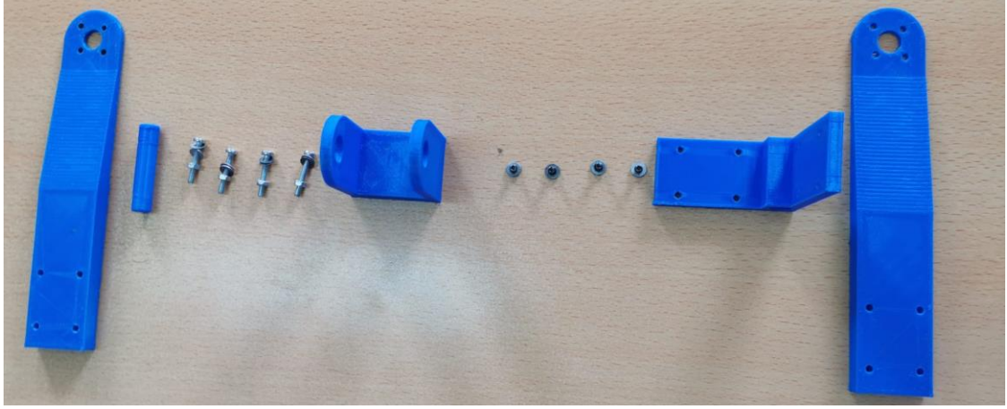
İtke Ölçme Sistemindeki Her Bir Parçanın Montaj Öncesi Görüntüsü
