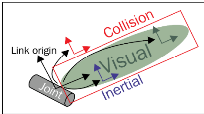
Şekil 29. URDF Uzun (link) ve Eklem (joint) Özellikleri Gösterimi ( http://wiki.ros.org/urdf/XML/link )
