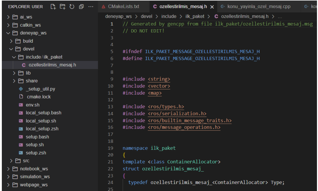
Şekil 16. ROS Tarafından Otomatik Olarak Oluşturulmuş Özelleştirilmiş Mesaj Başlık Dosyası
