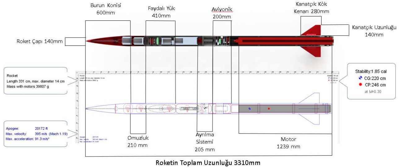
Şekil: Türkiye 2021 Teknofest Roket Yarışları Şampiyonu 1,5 Adana WOF Roketi Görünümü (Altta) ve Roket Kesit Görünümü (Üstte)
