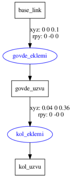
Resim 34. Robotun Uzun ve Eklem Hiyerarşisi
