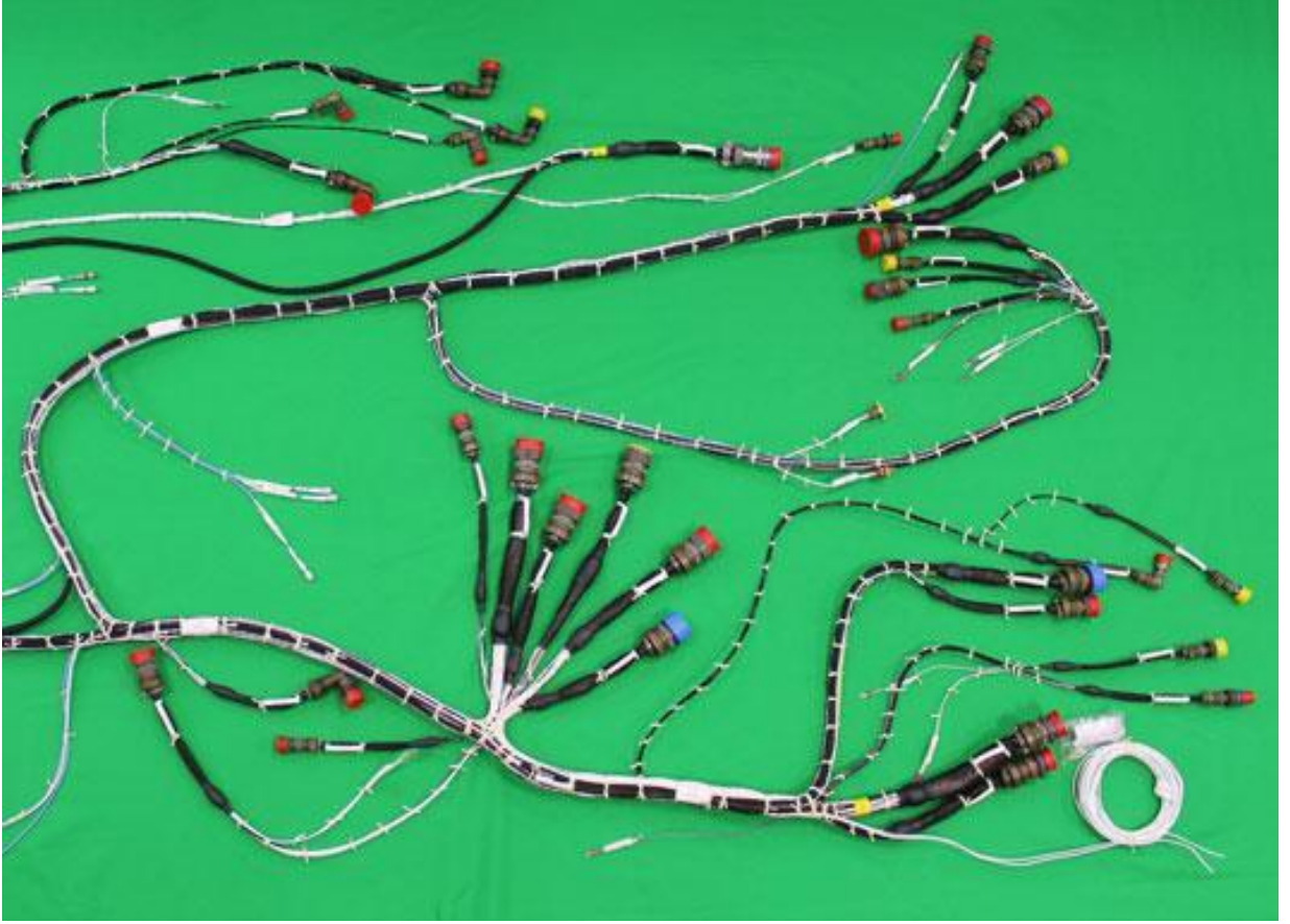
Şekil 6. Hava Araçlarında Kullanılan Konnektör ve Kablo Demeti Örnekleri
