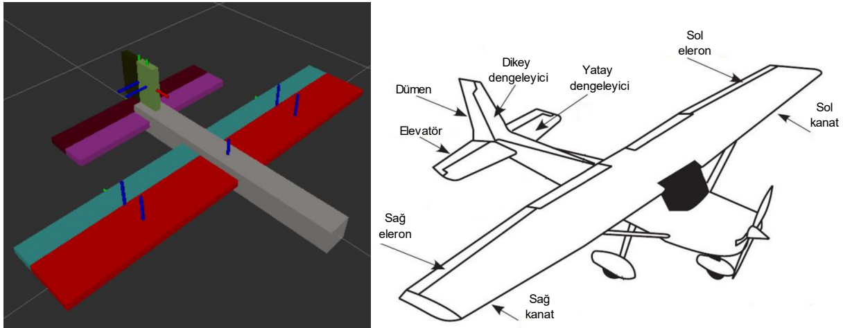
Şekil 39. Sabit Kanat Bir Uçağın Temel Sabit ve Hareketli Uzuyları ( https://core.ac.uk/download/pdf/43637015.pdf )
