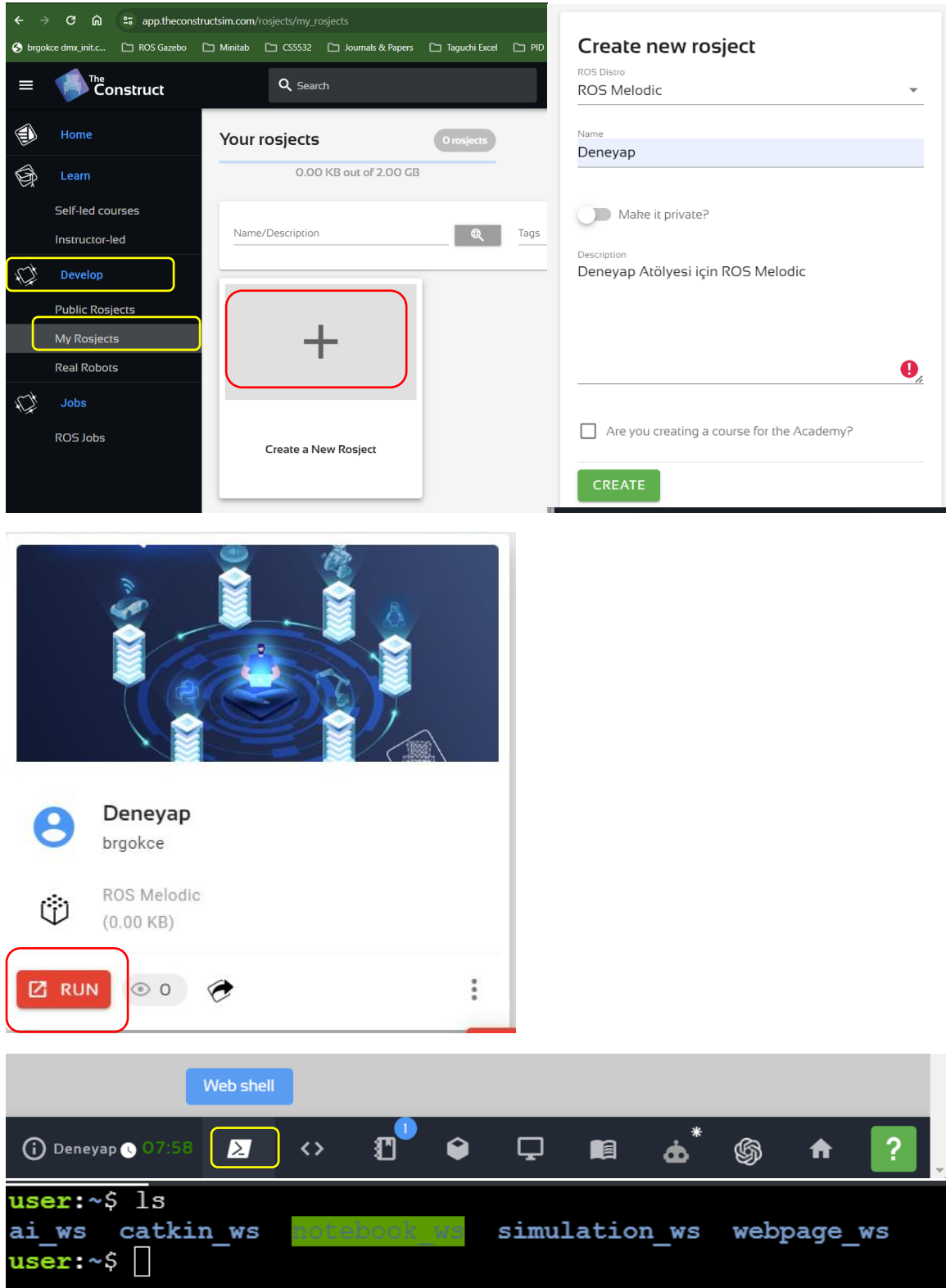
Şekil 1. theconstructsim.com Sistemindeki catkin_ws Çalışma Alanı
