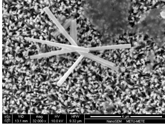
Çinko oksit nano çubuk kaplı cam yüzey
