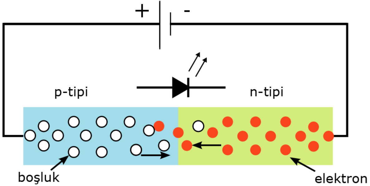
Yarı iletken bir LED'in şematik gösterimi. [ https://commons.wikimedia.org/wiki/File:PnJunction-LED-E.png ]
