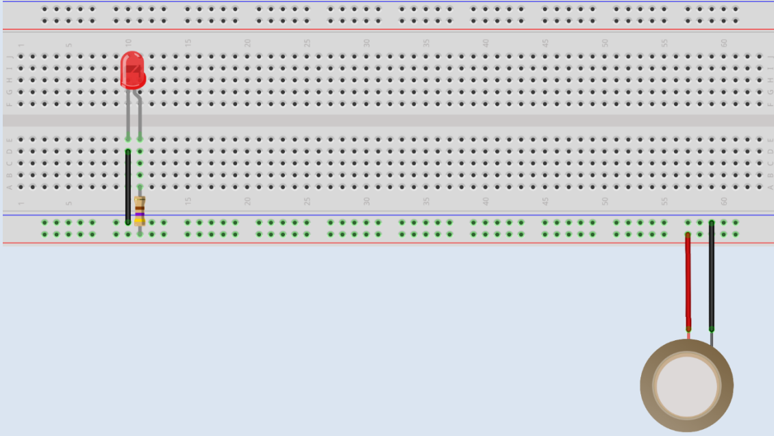
Deneyde kullanılacak olan devre tasarımı
