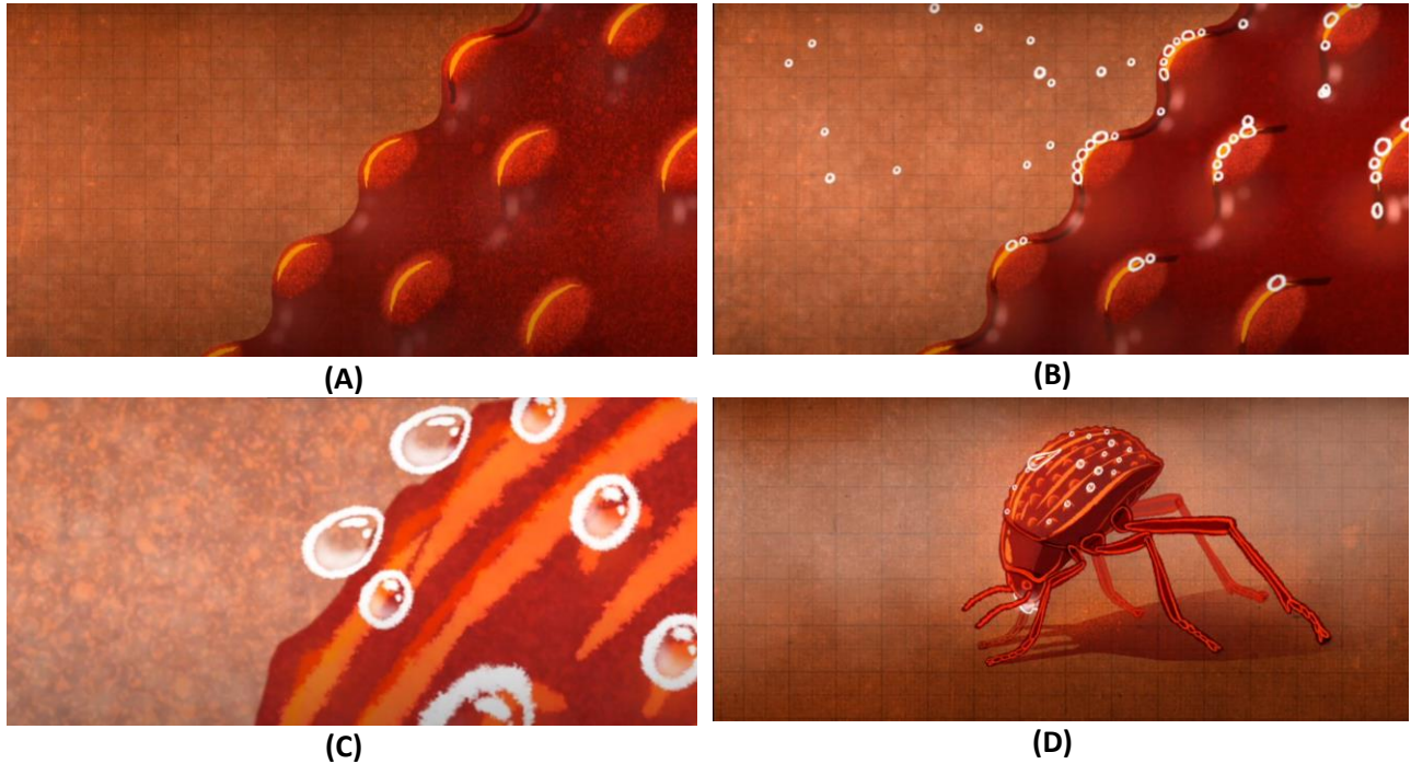
Namib çöl böceği kabuğu üzerinde sis'in içelebilir suya dönüşmesi. [BBC World Service Youtube Kanalı: https://youtu.be/OCBS6cjgYFM ]
