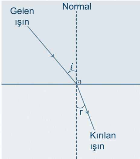
Bir ışığın bir ortamdan başka bir ortama geçerken yaşadığı kırılmanın illüstrasyonu.
