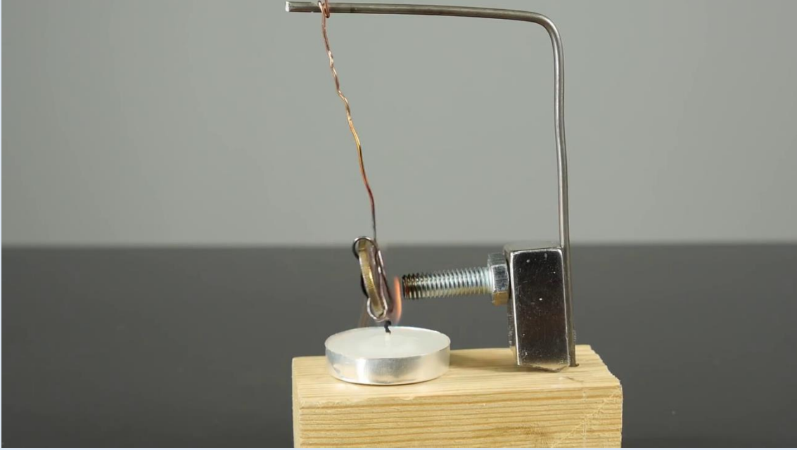
Soğuyan nikel parçanın tekrardan mıknatıs tarafından çekilmesi Kaynak: https://www.youtube.com/watch?v=h-FP9TmDAk0
