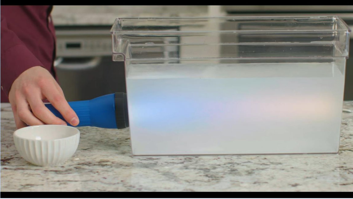
Su ve süt karışımına fenerle aydınlatılması sonucu oluşam mavi ve sarı bölgeler.
